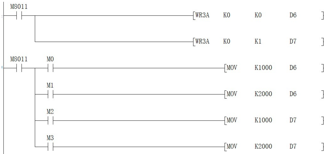
图 4-8 模拟量输出程序例子
