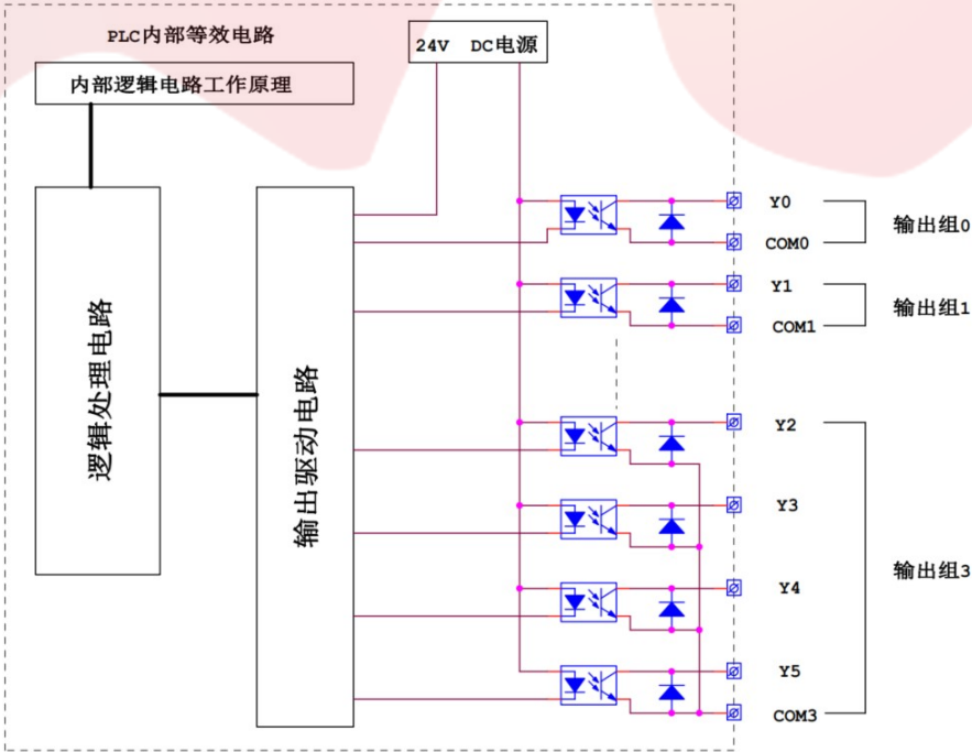
图 3—6 晶体管输出等效电路
