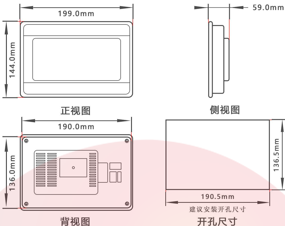
7 寸一体机安装尺寸图
