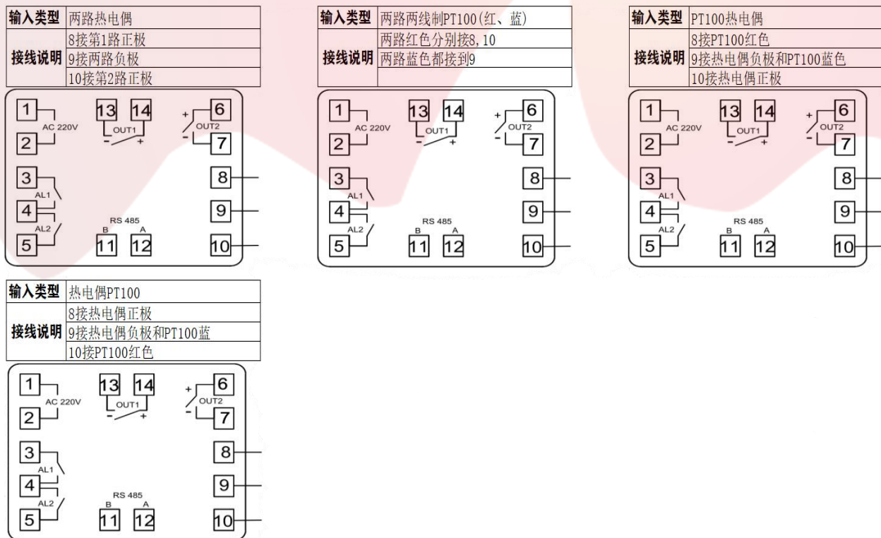
图 5-2 T02 接线图
