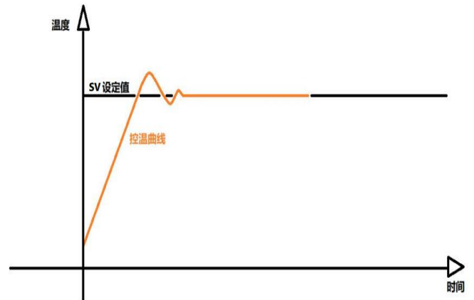
图 4-2 PID 控温曲线
