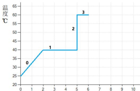
图 9-3-1 温度曲线
